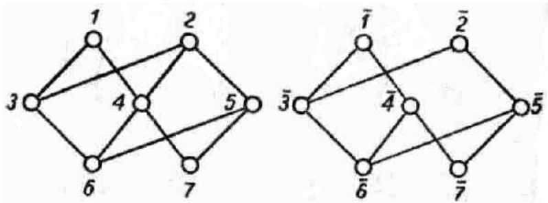
Рис. 8.7. Здесь изображены две частичные хронологии из двух описаний одного и того же набора событий 1, 2 ...7. Эти две хронологии различны, ибо второй источник (описанные в нем события имеют для различения черточку над их номером) не дает нам информации о временном соотношении событий 2 и 4. Разночтения в источниках могут быть и гораздо более серьезными вплоть до неразрешимых противоречий, приводящих к противоречащим друг другу частичным хронологиям.
