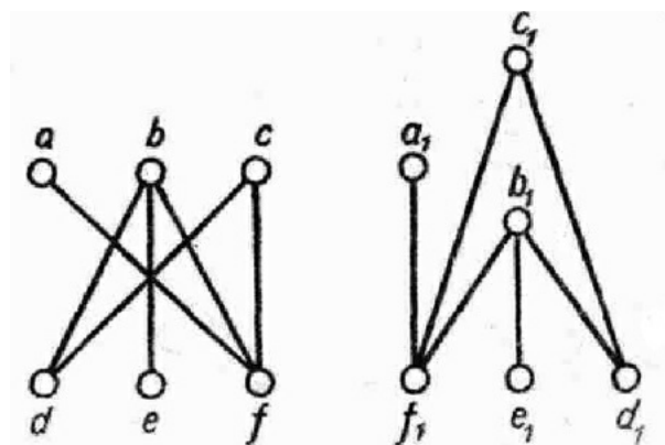
Рис. 8.6. При схематическом изображении частичных хронологий следует иметь в виду, что разные рисунки могут иногда представлять одинаковые хронологии, как, например, две изображенные здесь идентичные хронологии. В этом примере события a, b, c, d, e, f взяты из одного источника, а события a_1, b_1, c_1, f_1, e_1, d_1 являются описаниями тех же событий в другом источнике. Чтобы избежать такого рода недоразумений полезно пользоваться фиксированными картинками для всех типов хронологий, такими, как на рисунках 8.3, 8.4 и 8.5.
