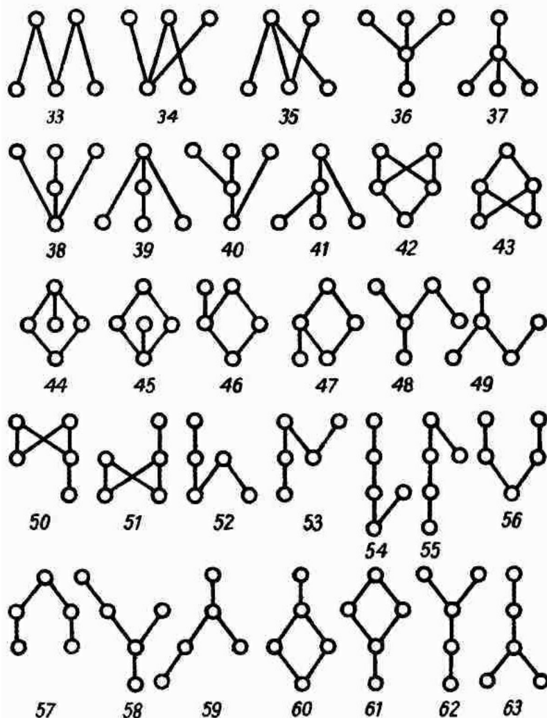
Рис. 8.5. Некоторые из возможных частичных временных упорядочений для множества, состоящего из пяти разных исторических событий. Про два события, которые не соединены на схеме черточкой или последовательностью ведущих вниз черточек, исторический источник умалчивает, которое из двух событий произошло раньше, а которое – позже. Для дальнейшей разработки этих хронологий нужно привлекать информацию из дополнительных источников, если таковые существуют. При этом нужно следить за тем, чтобы новая информация не была в противоречии со старой.
