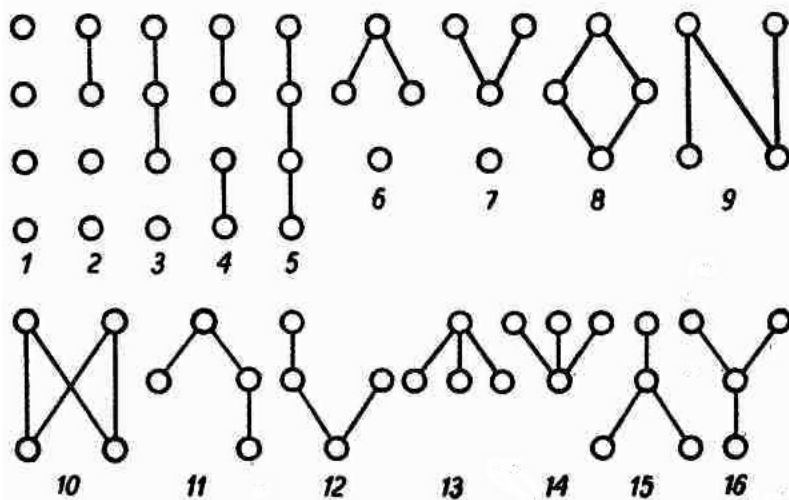
Рис. 8.4. В случае четырех событий из источника может следовать хронология одного из изображенных здесь типов. В каждом из типов возможны разные привязки к временной оси (датировки отдельных событий). В этом смысле количество возможных хронологий для четырех событий возрастает еще больше. Поэтому любимая историками хронология с точной датировкой всех событий является редчайшим исключением из правила и должна быть каждый раз тщательно обоснована.
