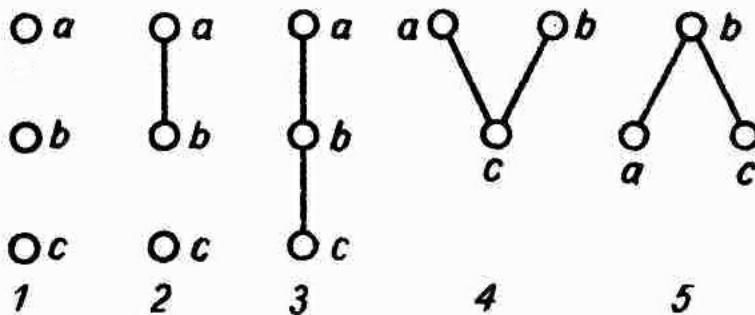
Рис. 8.3. Если в хронике упомянуты три исторических события, происшедшие в разное время, то их временное упорядочение по принципу «раньше-позже» может иметь один из пяти типов: 1. Никакой временной информации. 2. Одно событие произошло позже другого, но о времени третьего события ничего не известно. 3. Множество событий линейно упорядочено (возможны шесть разных таких упорядочений). 4; Два события произошли позже третьего, но неизвестно, как они соотносятся между собой. 5. Два события произошли раньше третьего, но неизвестно, как они соотносятся между собой. Здесь расположенные выше события считаются происшедшими позже.
